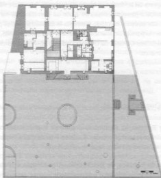
Planta do rés-do-chão e do jardim.
